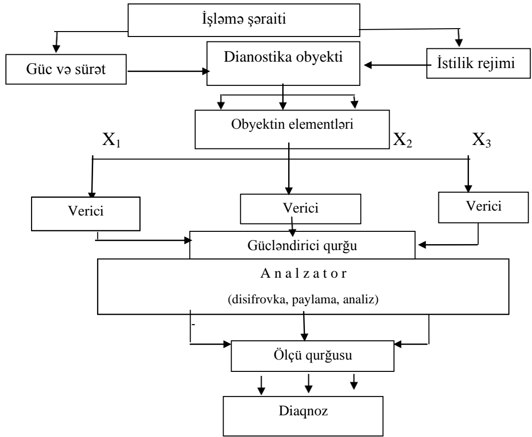
Şəkil 6. Diaqnostika prosesinin sxemi
