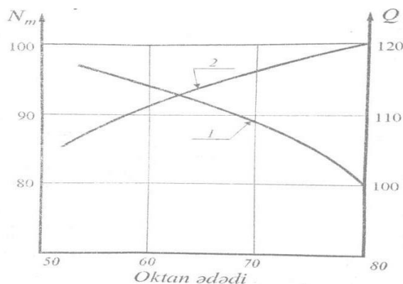
Şəkil 3. Gücün ( N_m ) və yanacaq sərfinin ( Q ) oktan ədədindən asılılıq əyriyə.
