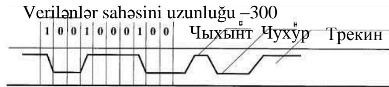
CD-ROM cığırının profili
