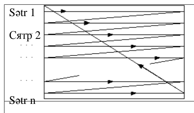
Elektron dəstəsinin ekranda hərəkəti
